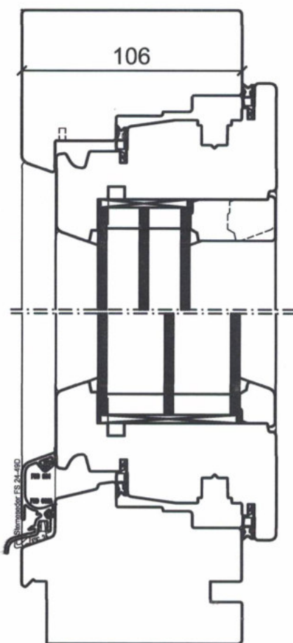
Rejet d'eau aluminium
