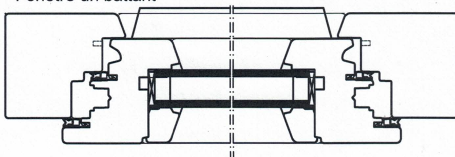
Fenêtre un battant
