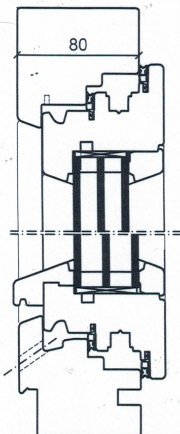
Traverse basse bois
