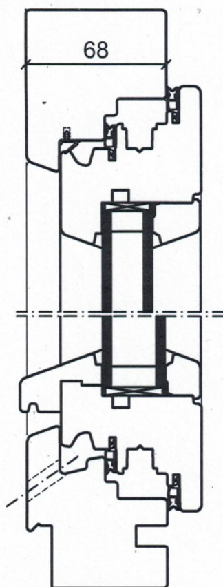
Traverse basse bois
